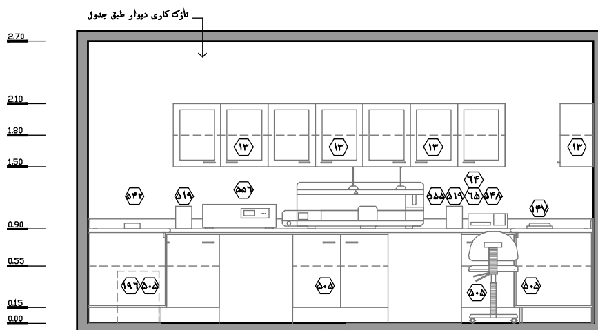
نقشه ۲-۴۷-۱۰ نمای ۱۰- مقیاس ۱:۵۰
