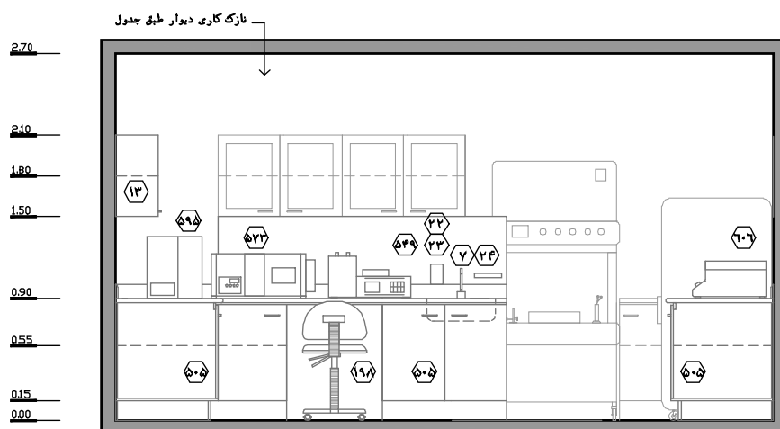
نقشه ۲-۴۶-۹ نمای ۹- مقیاس ۱:۵۰
