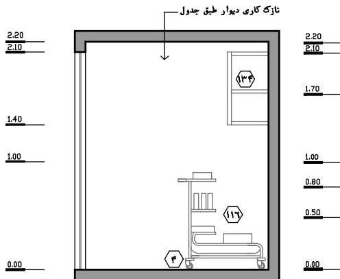
نقشه ۲-۸۶- نمای ۳- مقیاس ۱:۵۰
