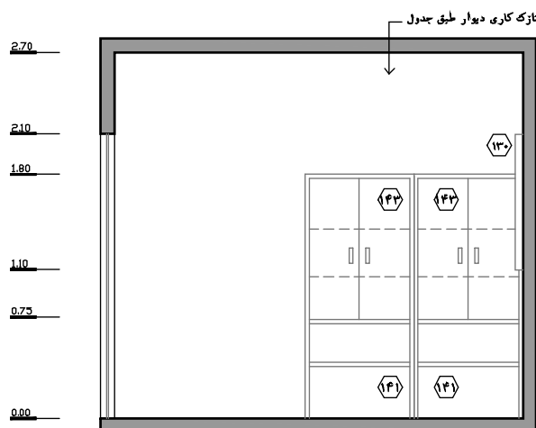
نقشه ۲-۷-۱ نمای ۱- مقیاس ۱:۵۰
