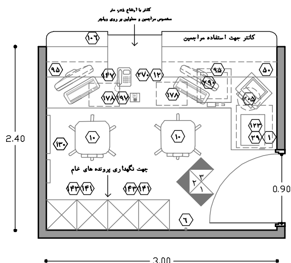
نقشه ۲-۶-۱ پلان نمونه‌ی پذیرش، صندوق، جوابدهی - مقیاس ۱:۵۰
